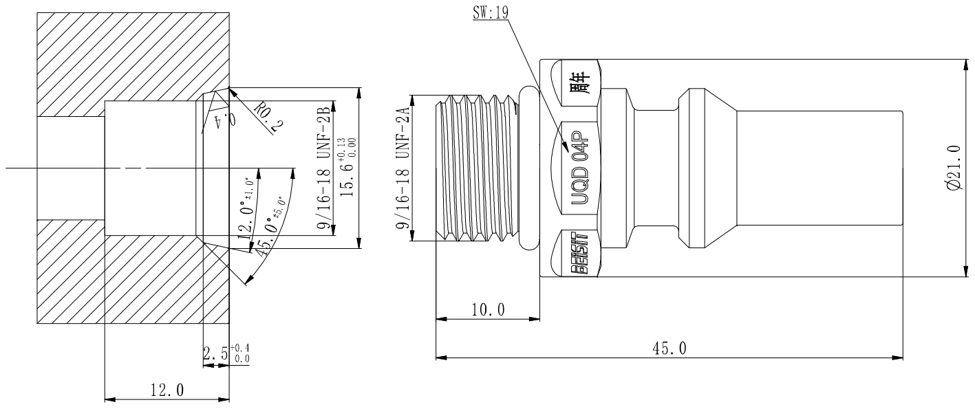
开孔尺寸
